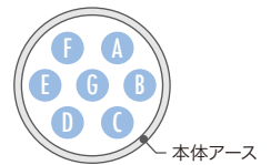
図2 プリアンプコネクタ(例)
