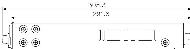
側面図
